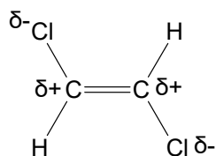
E -1,2-dichloroethene
