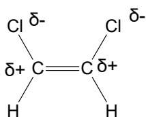
Z -1,2-dichloroethene
