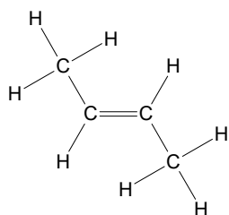
E-but-2-ene
