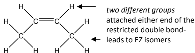
Z-but-2-ene
